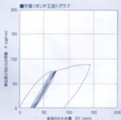
図-1.2 荷重と全体の たわみ量との関係 (試験体 No.2)
