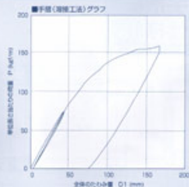
図-1.1 荷重と全体の たわみ量との関係 (試験体 No.1)
