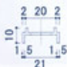
格子用チャンネル (A-3142)
