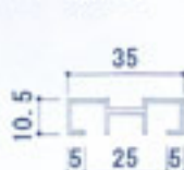
パーティションW材押え (K-11150)
