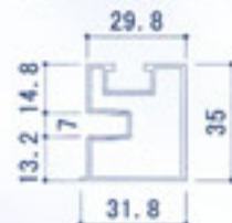
パーティションH材 (K-12011)
