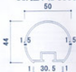
50丸笠木 (B-5955)
