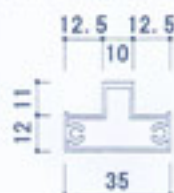
パーティションW材 (K-11152)
