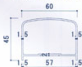
笠木一体型 (B-6394)
