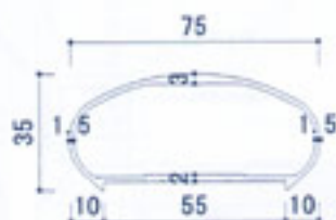
楕円笠木 (B-6883)
